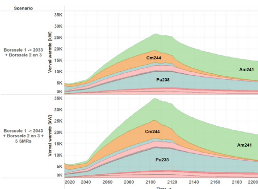
Verval warmte Warmte productie per isotoop, per scenario.
