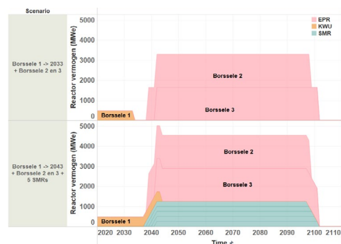
Reactorpark Evolutie van het opgesteld vermogen voor de twee beschouwde scenario's.
